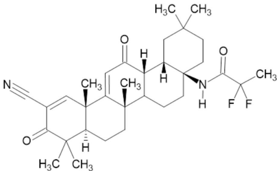
Rycina 1. Struktura chemiczna omaweloksolonu ( N -[(4 a R,6 a R,6 b S,12 a S,14 a R,14 b R)-11-cyano-2,2,6 a ,6 b ,9,9,12 a -heptametylo-10,14-dioksa-1,3,4,5,6,7,8,8 a ,14 a ,14 b -dekahydropicen-4 a -ylo]-2,2-difluoropropanamid) Figure 1. Chemical structure of omeveloxolone ( N -[(4 a R,6 a R,6 b S,12 a S,14 a R,14 b R)-11-cyano-2,2,6 a ,6 b ,9,9,12 a -heptamethyl-10,14-dioxo-1,3,4,5,6,7,8,8 a ,14 a ,14 b -decahydropicen-4 a -yl]-2,2-difluoropropanamide)
